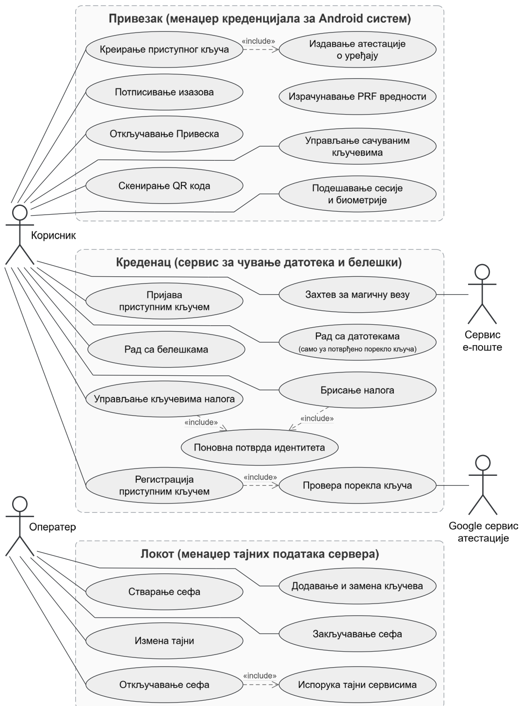
Слика 7: Случајеви коришћења система.
