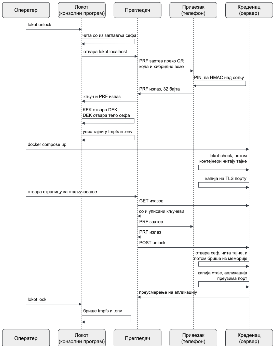
Слика 9: Ток покретања система.
