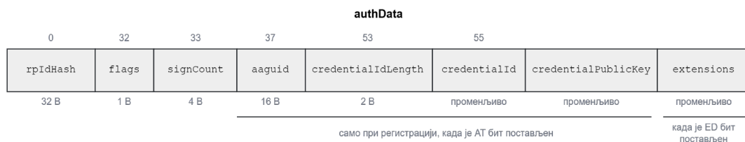
Слика 4: Структура authData записа.
