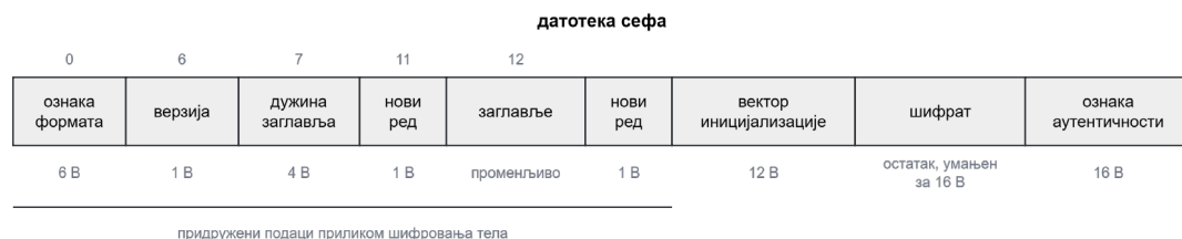
Слика 16: Распоред датотеке сефа.
