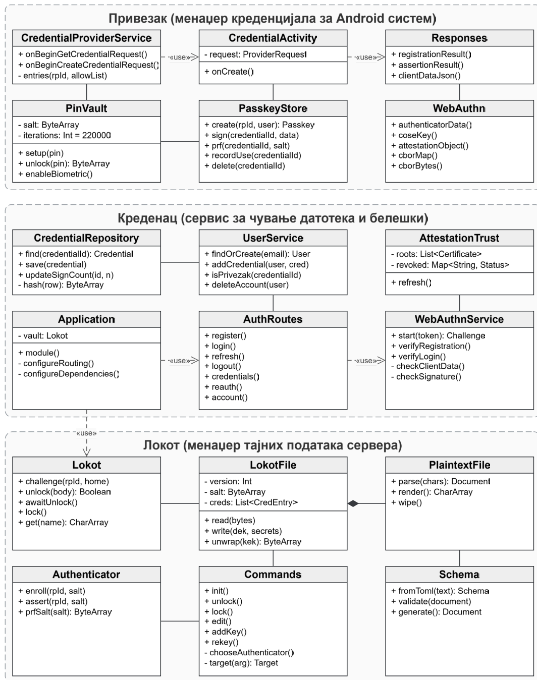
Слика 8: Упрошћени дијаграм класа три подсистема.
