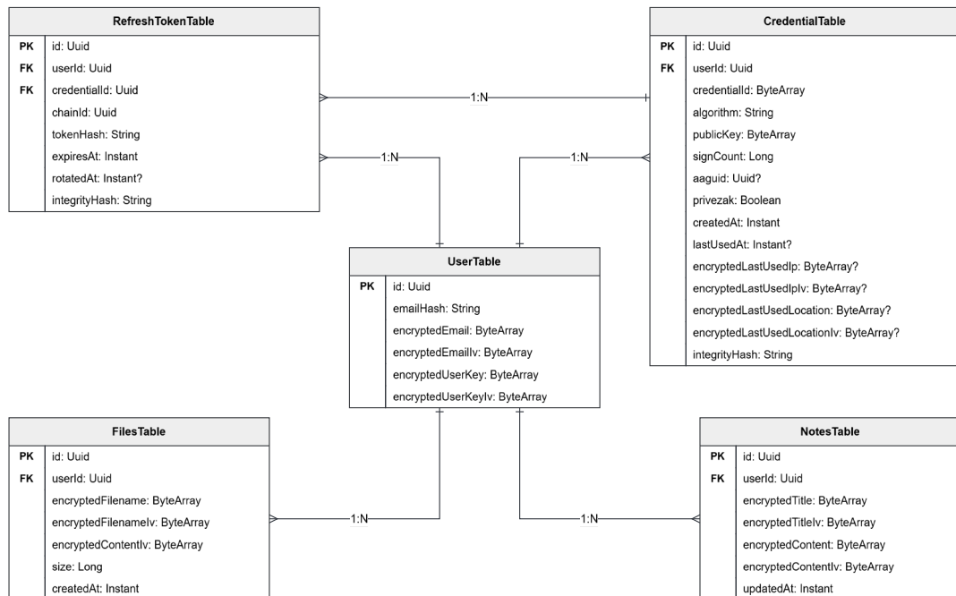
Слика 13: Модел података Креденца.
