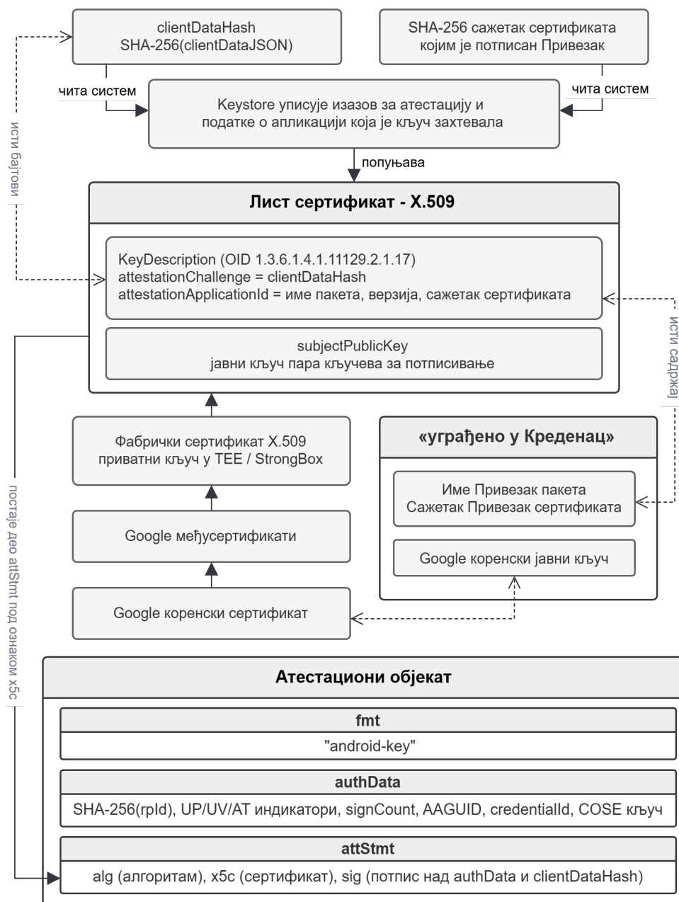
Слика 12: Настанак атестације и ланац сертификата.
