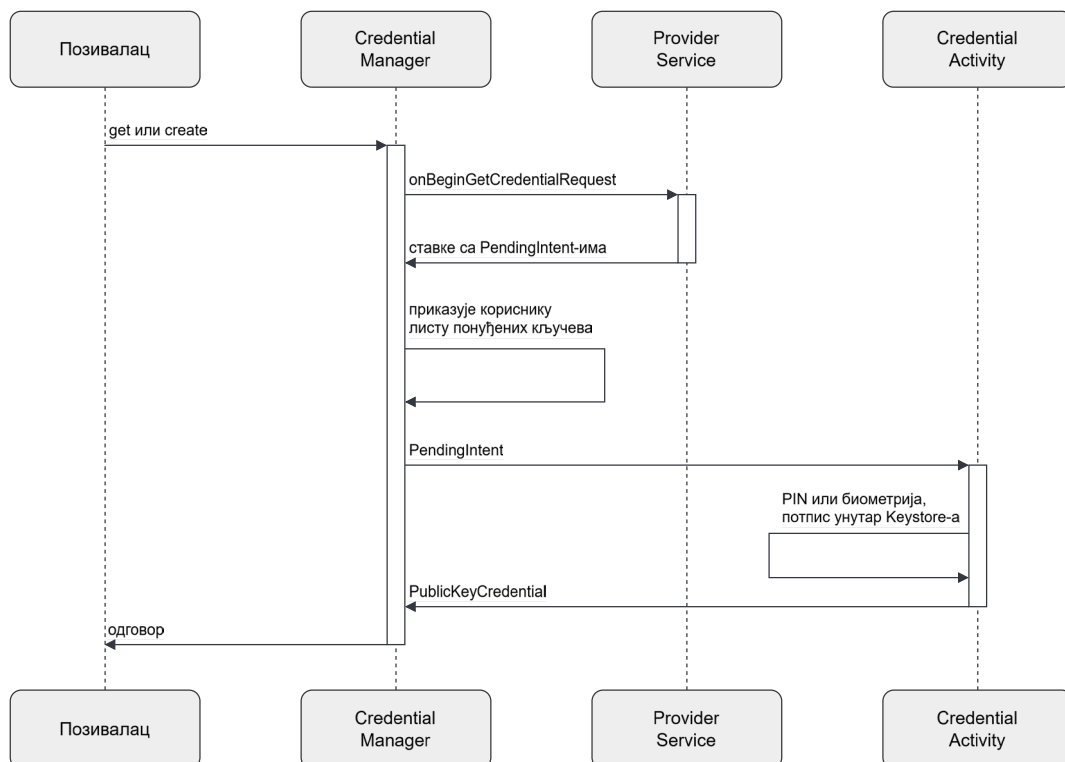
Слика 10: Ток обраде захтева у Привеску.
