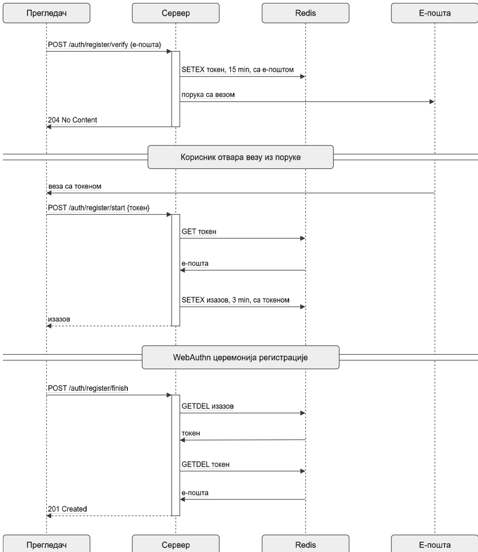
Слика 14: Ток регистрације магичном везом.
