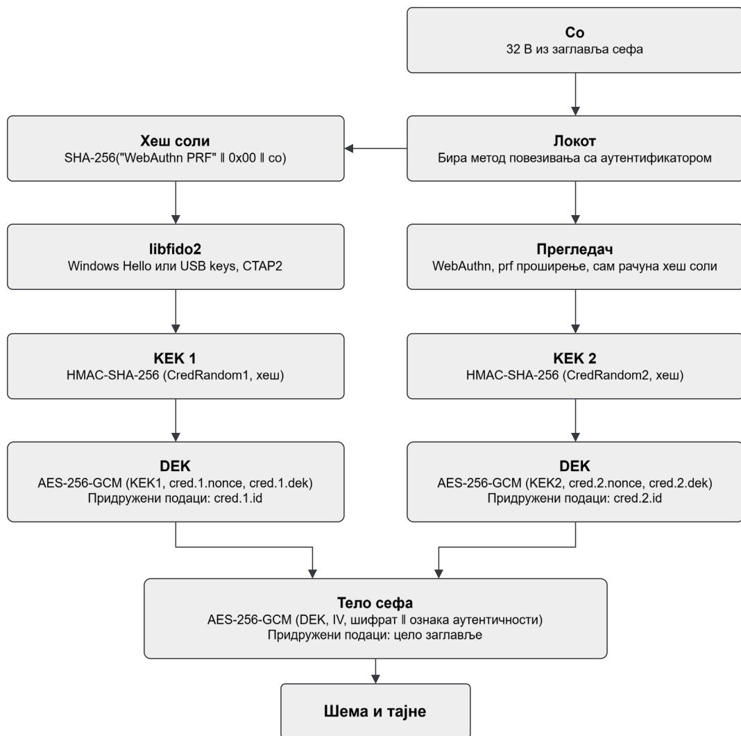
Слика 15: Пут од приступног кључа до тајни у сефу.
