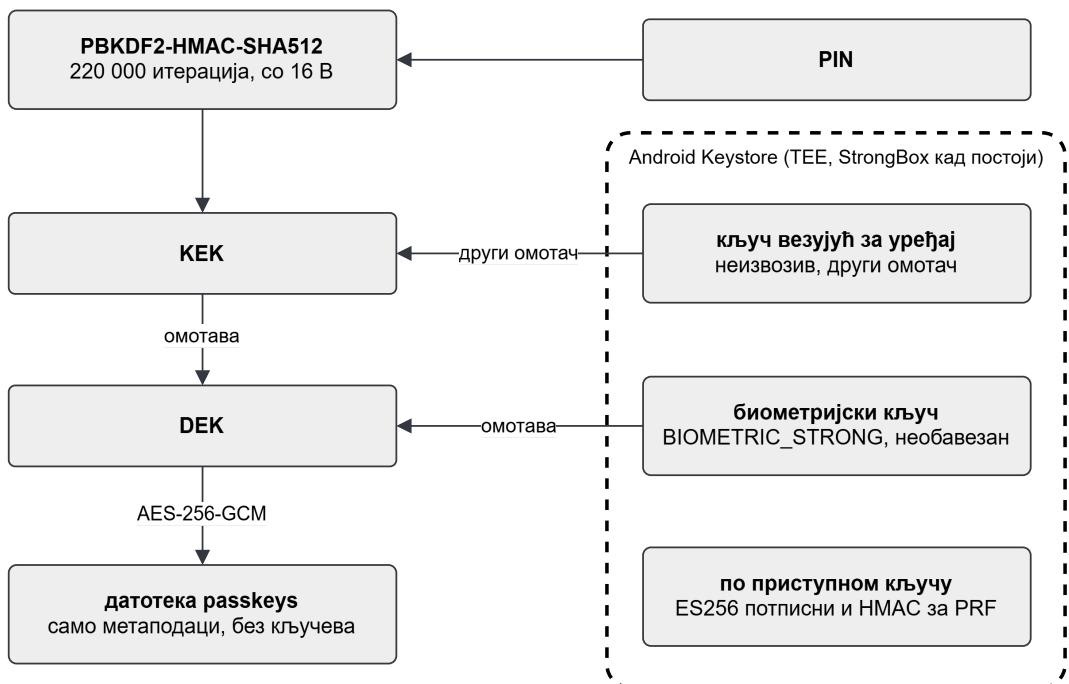
Слика 11: Хијерархија кључева у Привеску.
